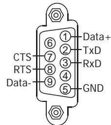
COM3: RS-232/RS-485
