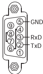
COM1: RS-232
