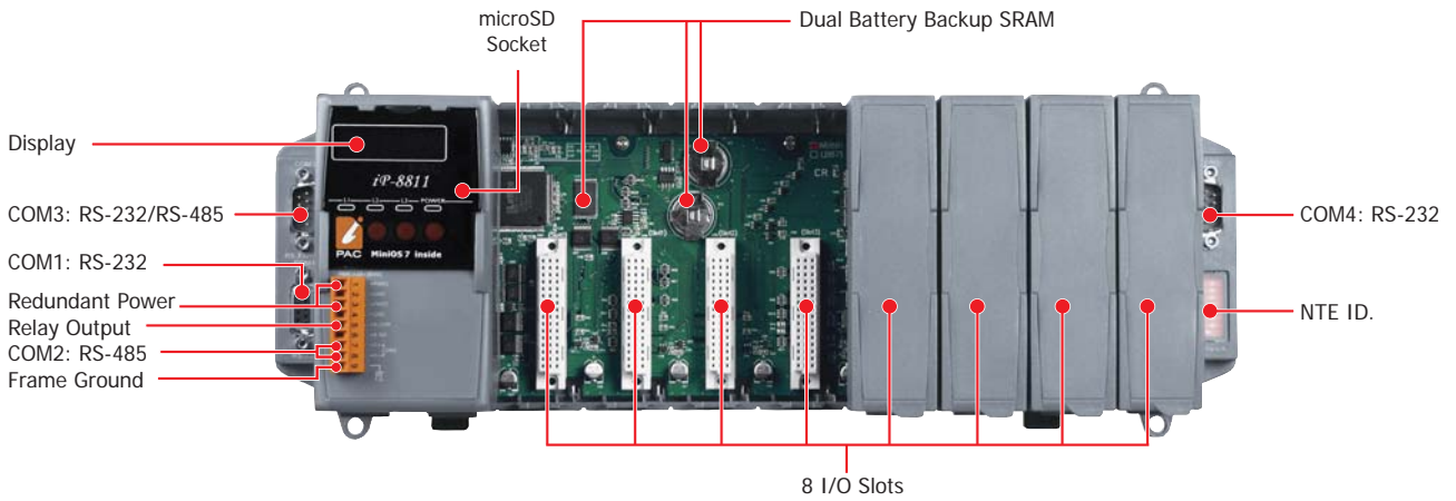
iP-8811
